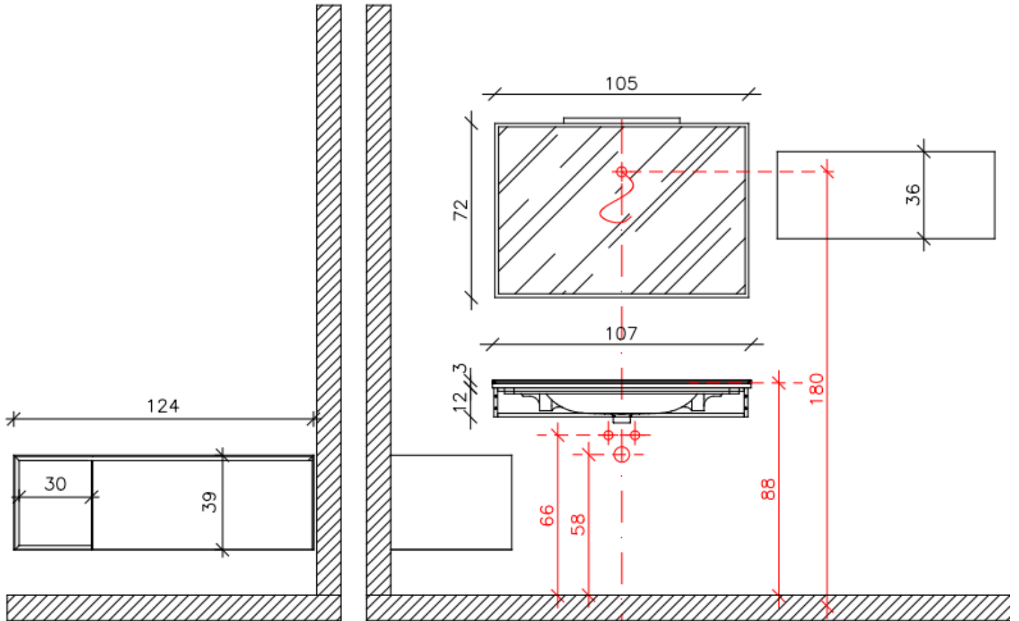
PROSPETTO
