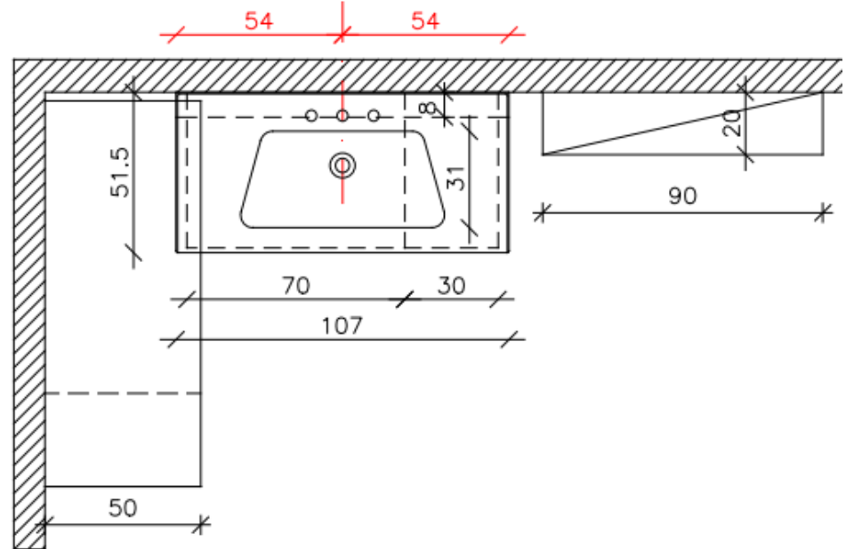
PIANTA
