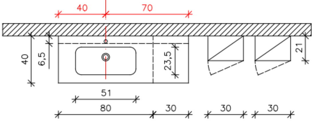
PROSPETTO
