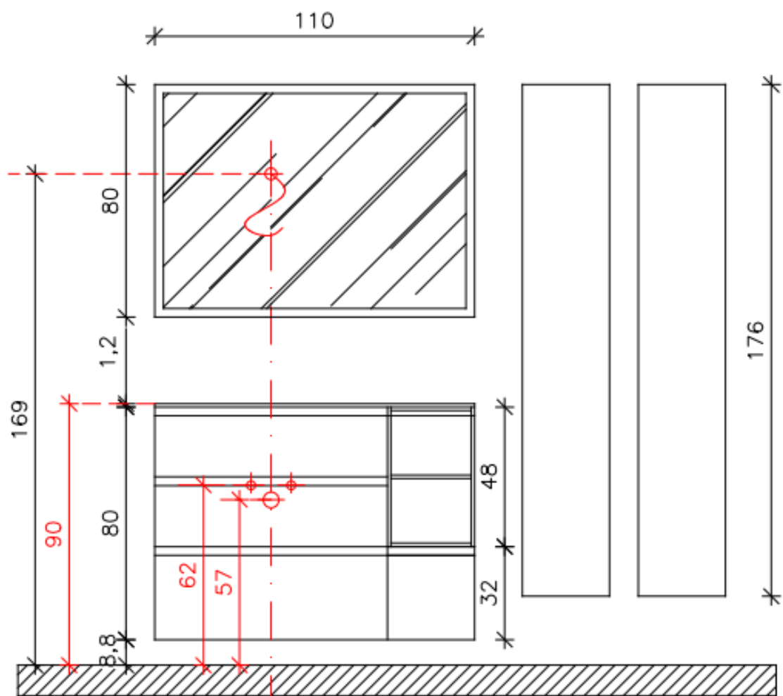
PROSPETTO
