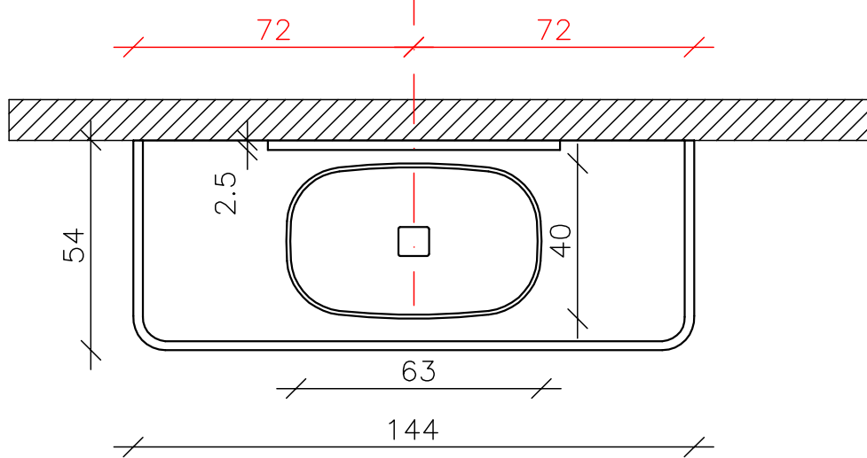
PIANTA
