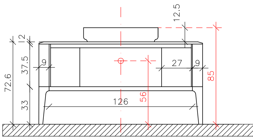
PROSPETTO
