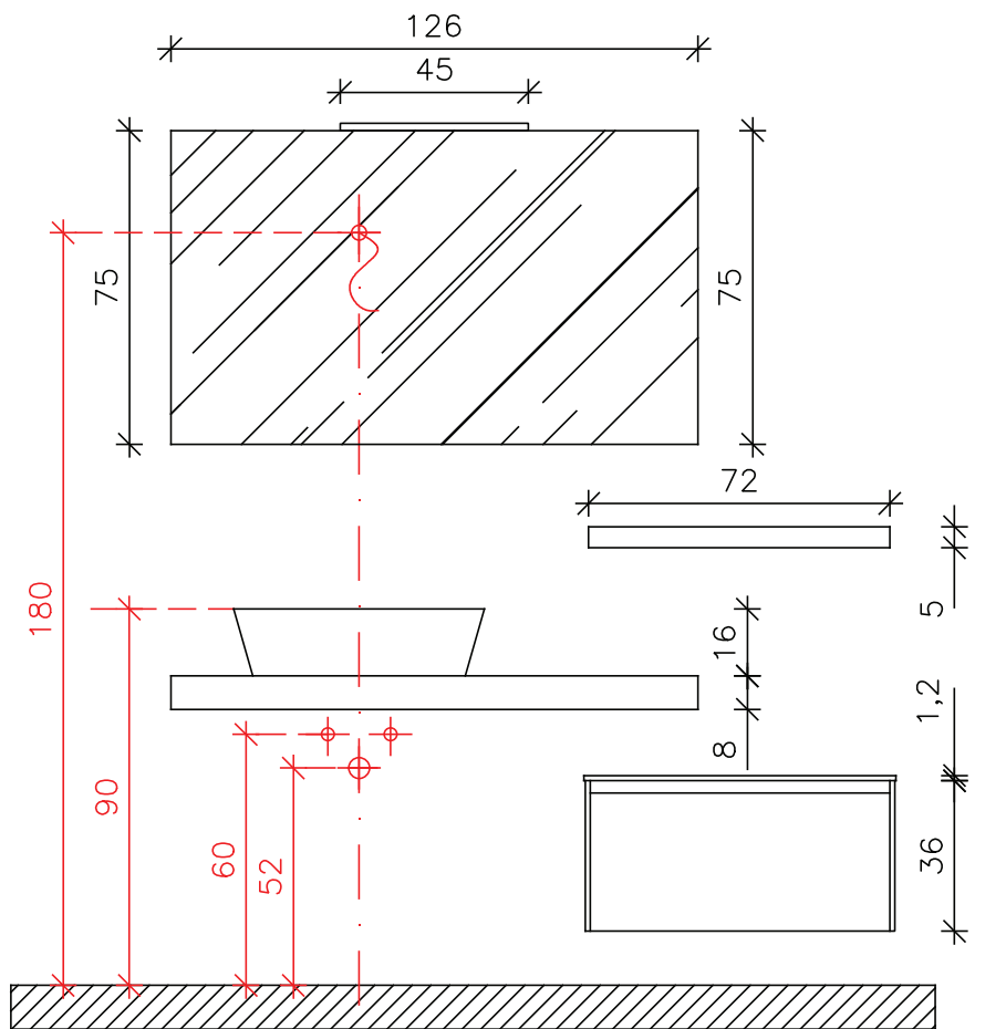
PROSPETTO
