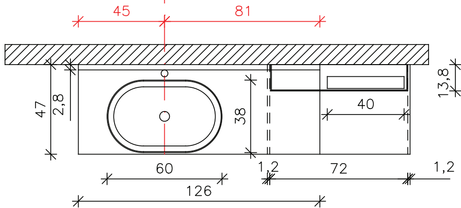
PROSPETTO
