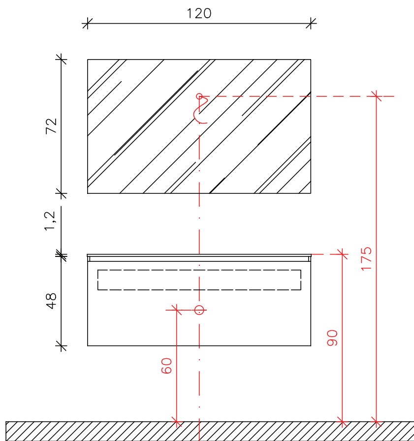
PROSPETTO
