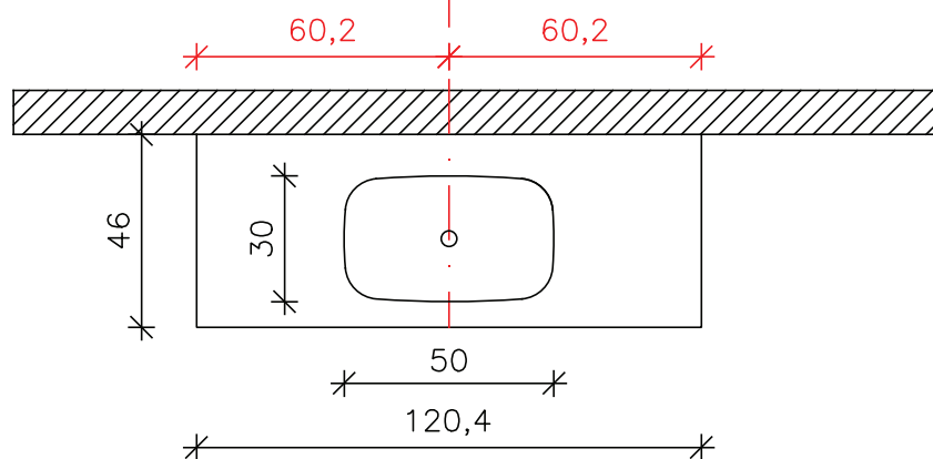
PIANTA
