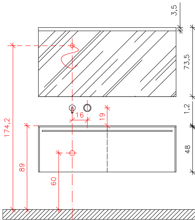
PROSPETTO
