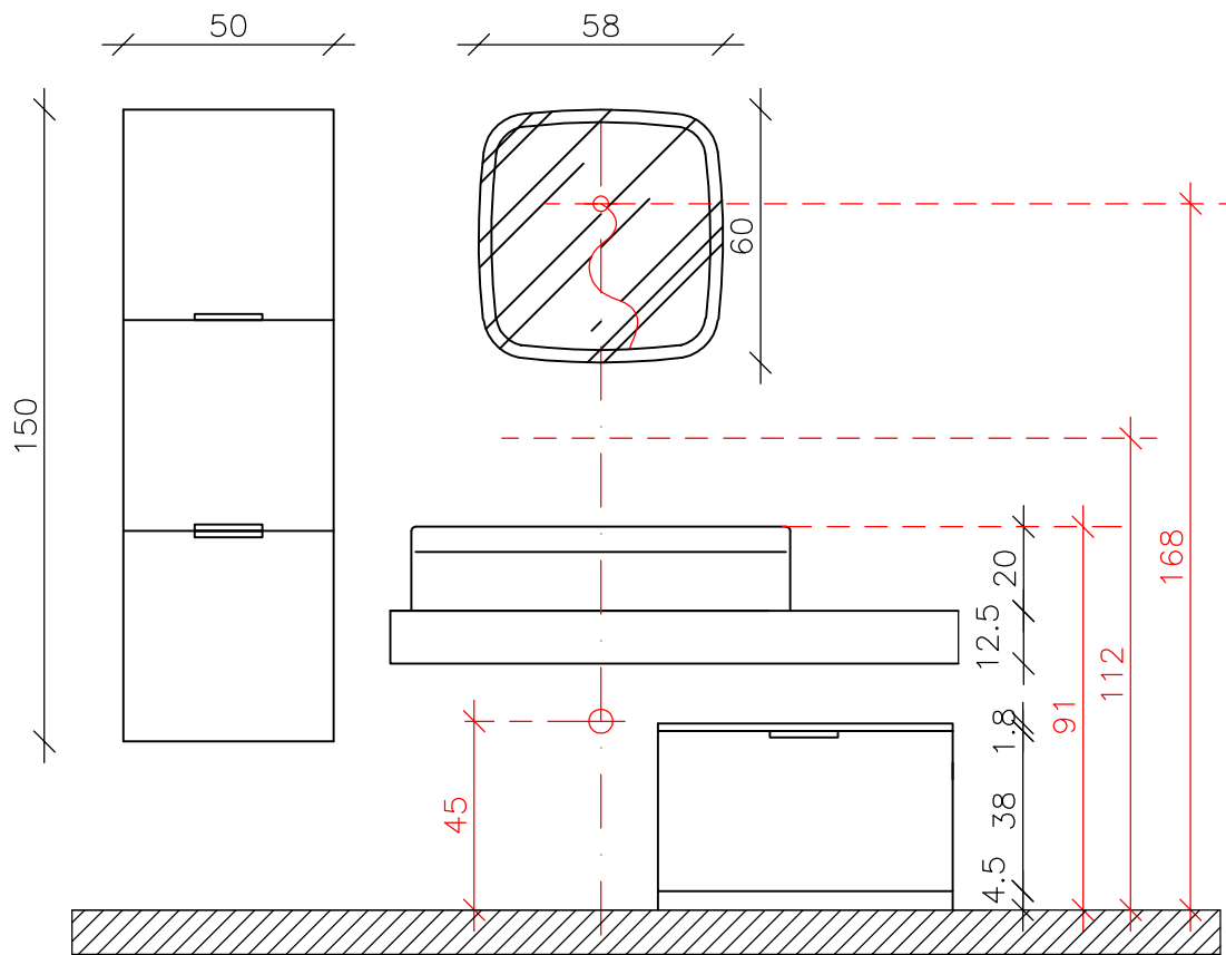
PROSPETTO
