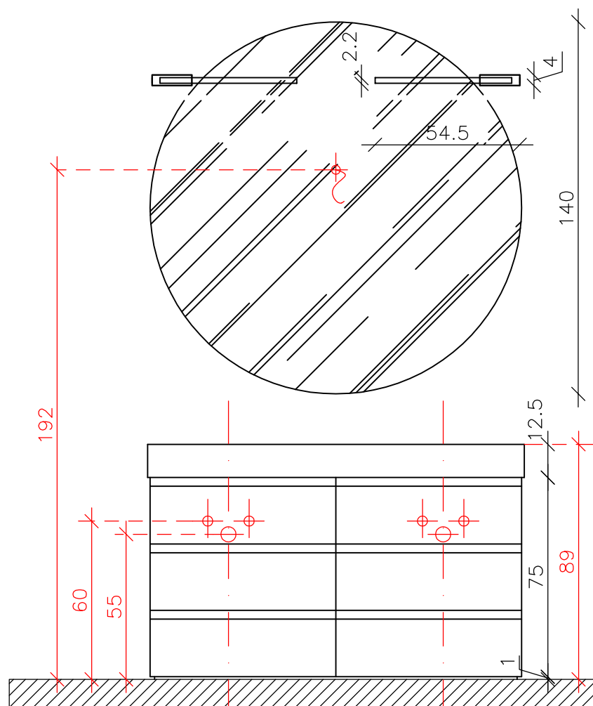
PROSPETTO
