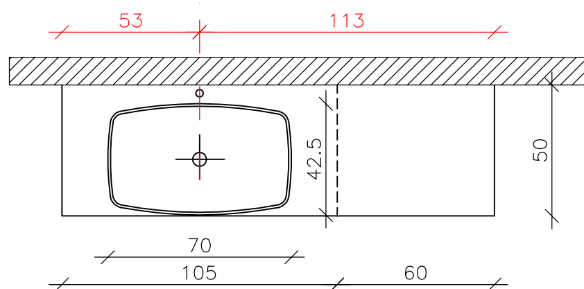
PIANTA
