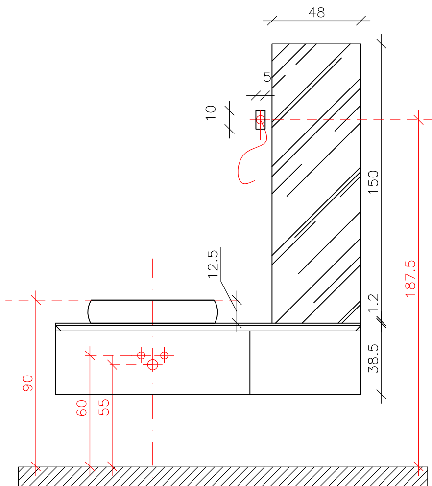
PROSPETTO
