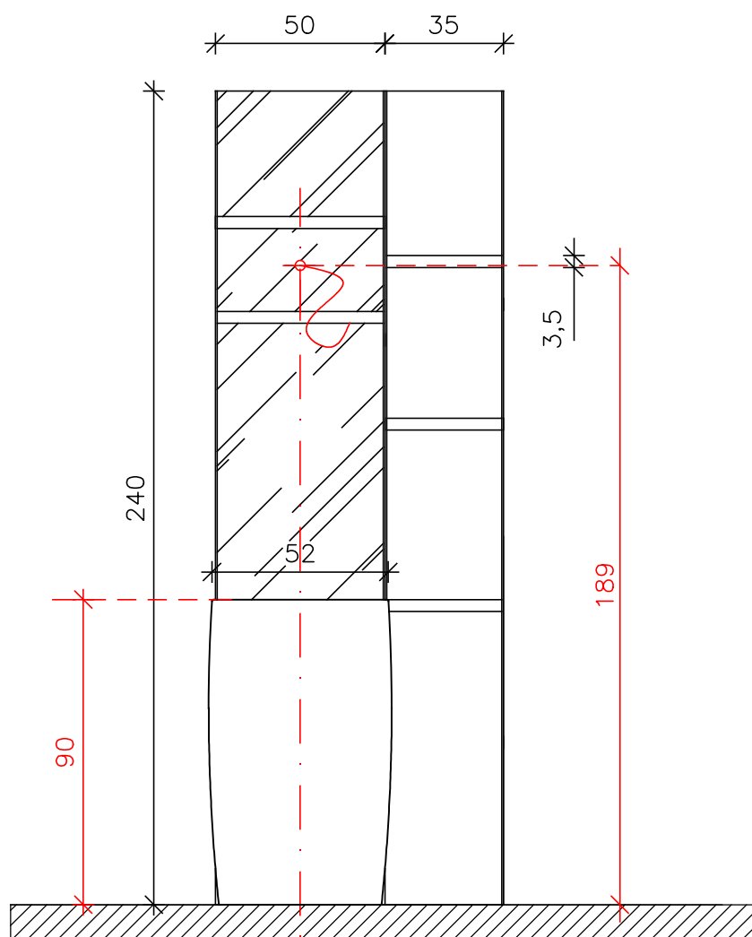
PROSPETTO
