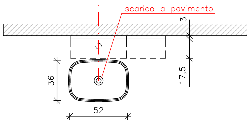
PIANTA
